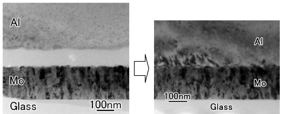
ガラスと金属の超音波接合過程
