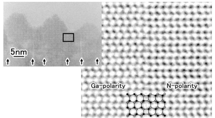
GaN 膜成長に発生する表面凹凸、貫通欠陥の成因解明 結晶成長面が数 nm 毎に変化することが原因と判明
