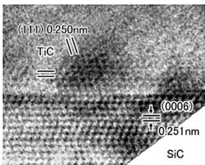
ロウ付けプロセスの原子レベルその場観察
